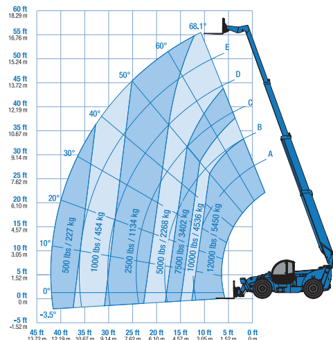
GTH-1256 | STABILISATEURS RELEVÉS
