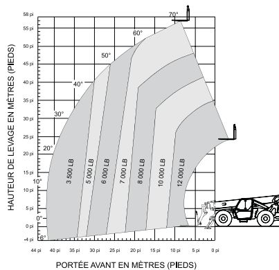
SJ1256 THS | STABILISATEURS ABAISSÉS
