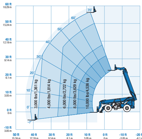
GTH-1056 | STABILISATEURS ABAISSÉS
