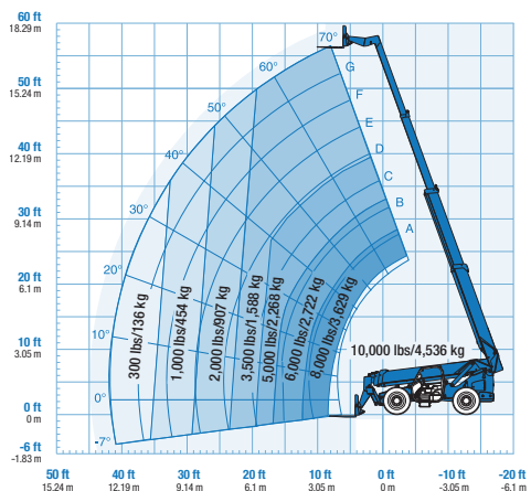
GTH-1056 | STABILISATEURS RELEVÉS
