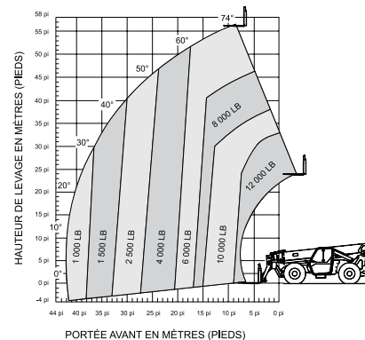
SJ1256 THS | STABILISATEURS RELEVÉS
