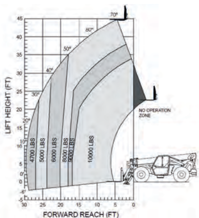
SJ1044 TH | STABILISATEURS ABAISSÉS
