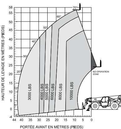
SJ1056 TH | STABILISATEURS ABAISSÉS
